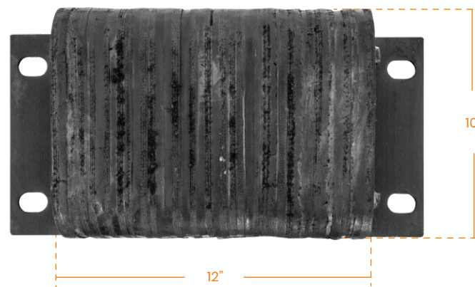
ANCHO Y ALTO Vista frontal
